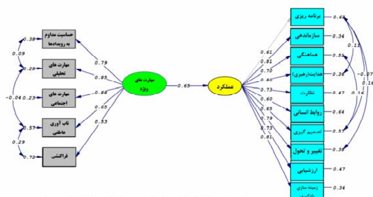
نمودار ۲: مدل معادلات ساختاری مهارت‌های ویژه خودباندگی و عملکرد (ضرایب مسیر)
